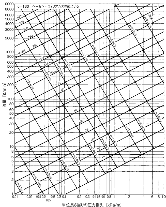
図16 硬質塩化ビニル管流量線図 (SHASE-S 206-2009)
