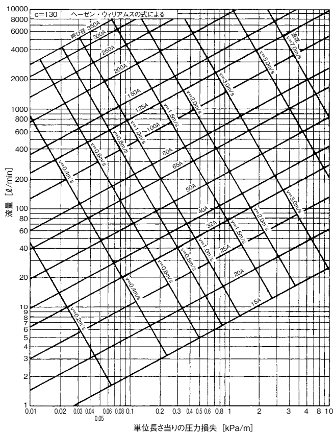
図17 硬質塩化ビニルライニング鋼管流量線図 (SHASE-S 206-2009)
