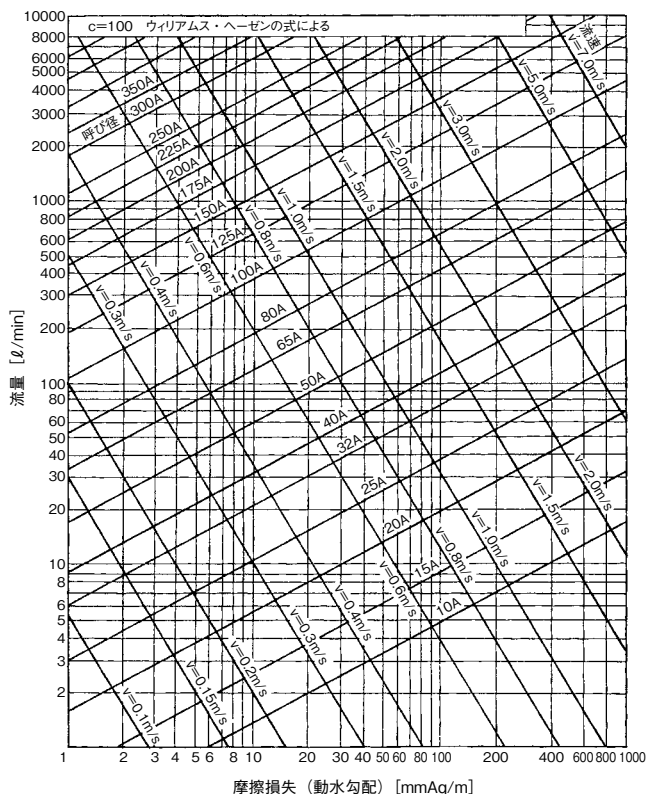
図14 配管用炭素鋼鋼管 (JIS G 3452) 流量線図 (HAS-S 206-1982)
