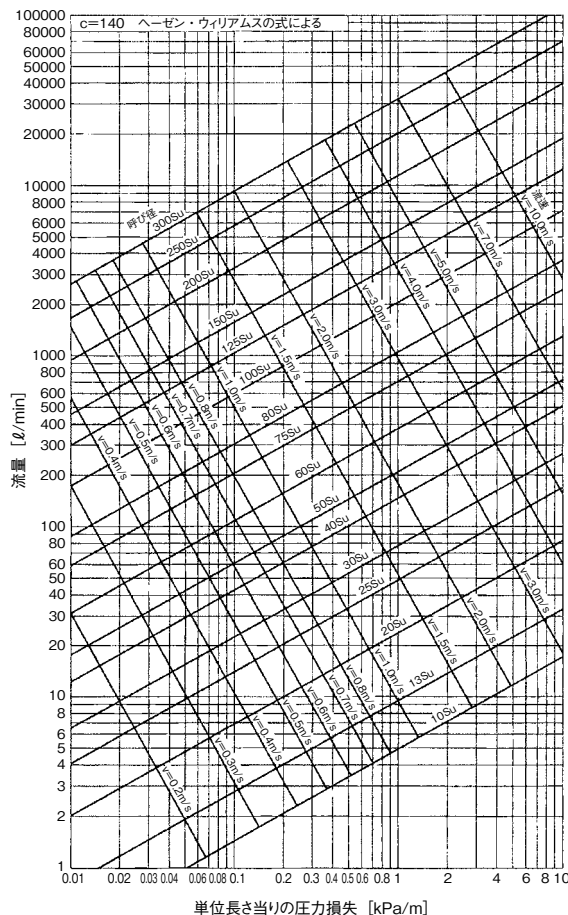
図15 一般配管用ステンレス鋼管流量線図 (SHASE-S 206-2009)
